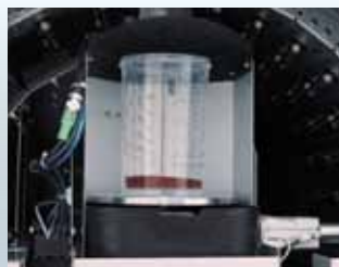
Präzisionswaage für Mischbecher von 50ml bis 2l
